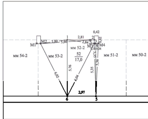
Фрагмент графической части проекта технического плана образуемого машино-места № 53-2
