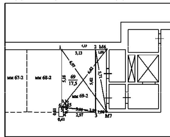
Фрагмент графической части проекта технического плана образуемого машино-места № 69-2
